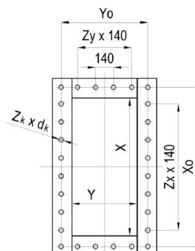
Kołnierz wylotu
