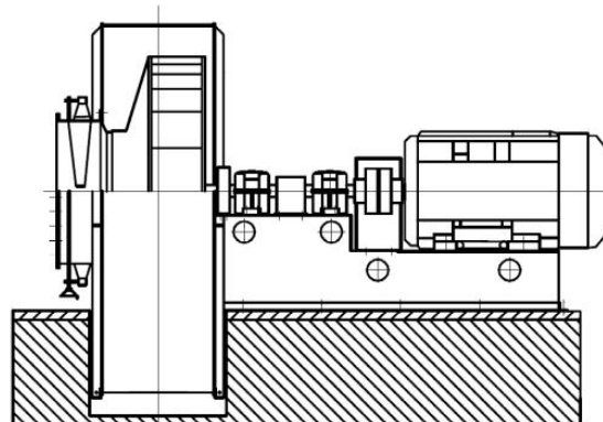
Wentylator promieniowy jednostrumieniowy z aparatem kierowniczym osiowym WP-/2,3 A
