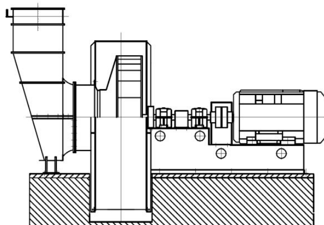
Wentylator promieniowy jednostrumieniowy z wlotem kolanowym i aparatem kierowniczym osiowym WP-/2,3 A
