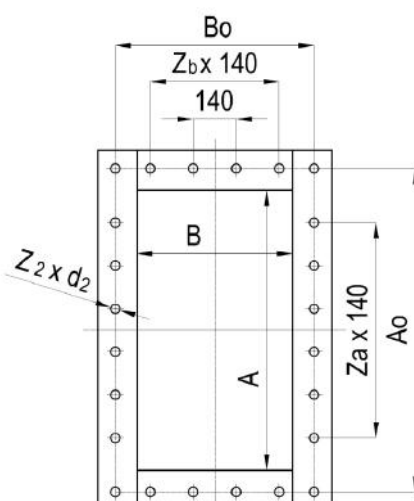
Kołnierz wlotu kolanowego
