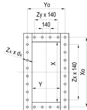
Kołnierz wylotu
