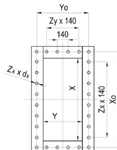
Kołnierz wylotu
