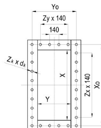
Kołnierz wylotu
